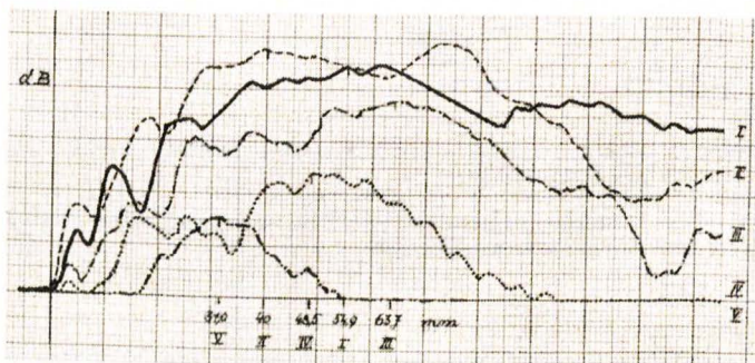
Abb. 14. Einschwingvorgang des offenen B 1 (58 Hz) Fig. 14. Attack transient of open B 1 (58 c/s)
