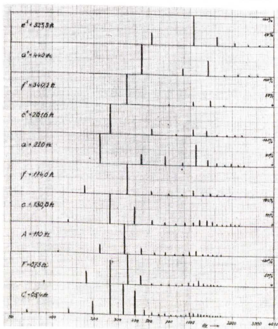
Tafel XII Klangspektren Luftschall — mit Dämpfer Plate XII Sound spectra Airborne sound — muted
