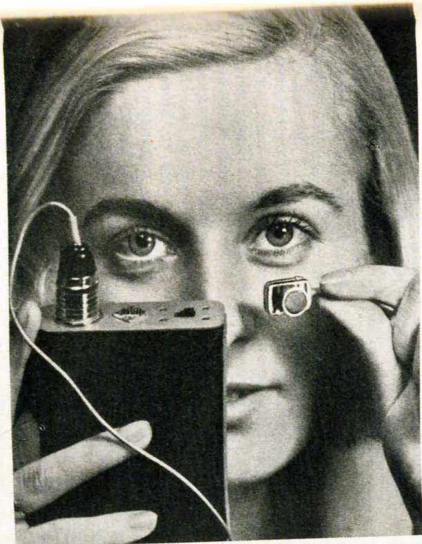
Transistortaschensender und Knopflochmikrofon der drahtlosen Mikrofonanlage Mikroport (Telefunken). Pocket transistor transmitter and buttonhole microphone of the Telefunken Mikroport.
