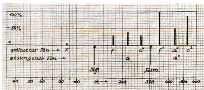
Abb. 19. Klangspektren des Doppeltones F—a^1 Fig. 19. Frequency spectra of the double note F—a^1
