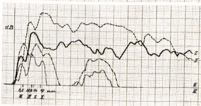
Abb. 15. Einschwingvorgänge des gestopften c' (270 Hz) a) sforzato angeblasen b) weich angeblasen Fig. 15. Attack of stopped c' (270 c/s) a) sforzato b) without accent
