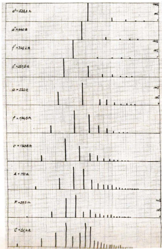
Tafel VI Klangspektren Luftschall — offen Plate VI Sound spectra Airborne sound — open
