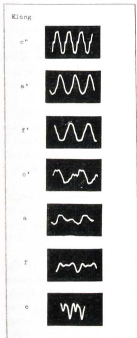
Tafel XI Oszillogramme gestopfter Töne (Luftschall, vergl. Tafel V)
