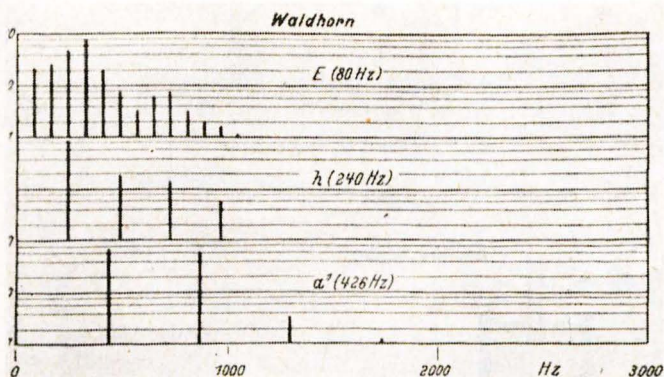
Abb. 99. Klangspektren eines Waldhorns. (Nach E. MEYER und G. BUCHMANN.)
