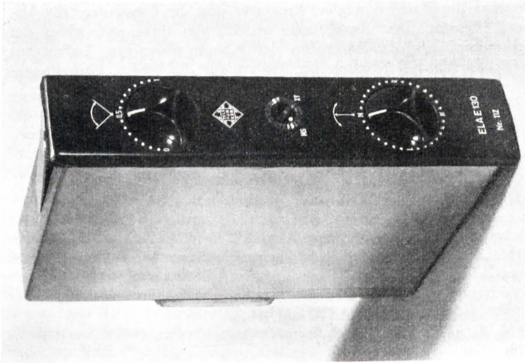
Bild 1 Stereo- Richtungsmischer Fig. 1. Stereo directional mixer.
