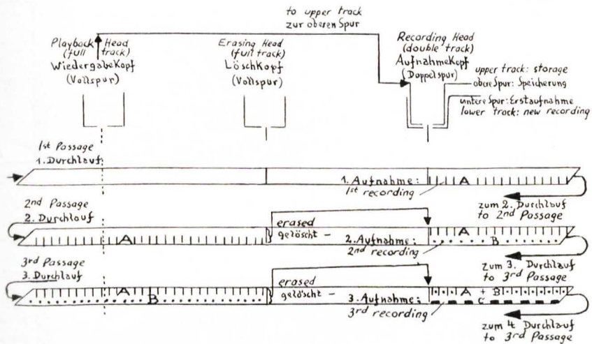
I. Spezialaufnahmeaggregat "System Heiss" - Schema des Aufnahmevorgangs I. Special recording unit "System Heiss" - Diagram of the recording process
