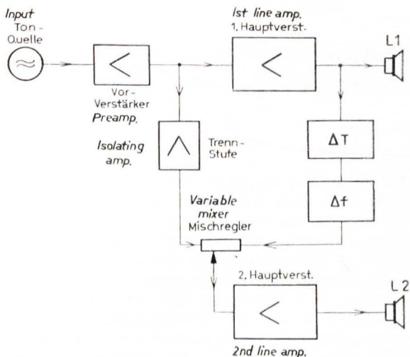
Abb. 2 Schema der Gewinnung eines pseudostereophonischen 2. Kanals durch Laufzeit- bzw. Halleinfluß ( \Delta T ) und Frequenzgangbeeinflussung ( \Delta f ) mit wählbarem Mischverhältnis zum 1. Kanal.
