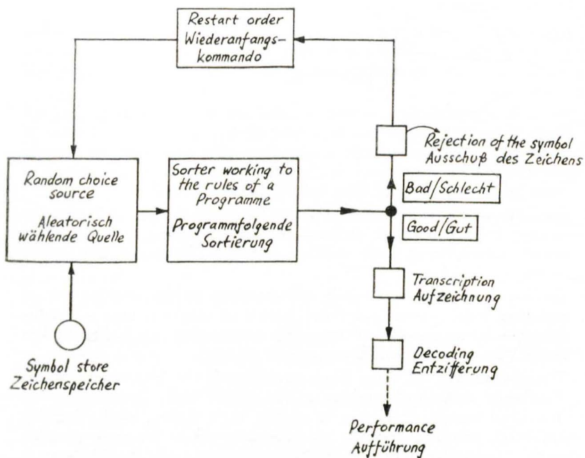
Abb. 11 Grundschemata eines musikalischen Kompositionsgerätes Fig. 11 Elementary block diagram of a musical composition machine
