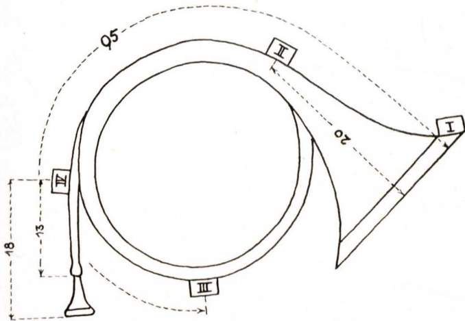
Abb. 12. Die Ansatzpunkte des Mikrophons (I—IV) zur Messung des Körperschalles
