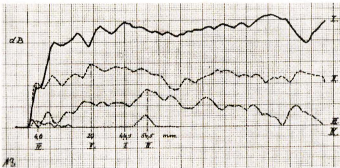
Abb. 13. Einschwingvorgang des offenen c^1 (268 Hz)
