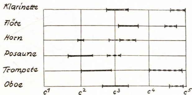
Hauptformant (—) Region Nebenformant (---) Region 1. Grades Nebenformant (····) Region 2. Grades Abb. 17. Formanten einiger Blasinstrumente
