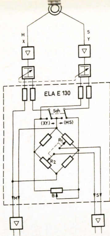
Schaltbild des Telefunken Richtungs-mischers ELA E 130, mit dem man eine feststehende Schallquelle elektronisch wandern lassen kann. Schematic of the Telefunken ELA E 130 Directional Mixer, by which the apparent position of a fixed sound source can be moved at will.
