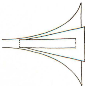
Abb. 18. Dämpfer im Schallbecher (Schnitt) Fig. 18. Sectional view of a mute in the bell
