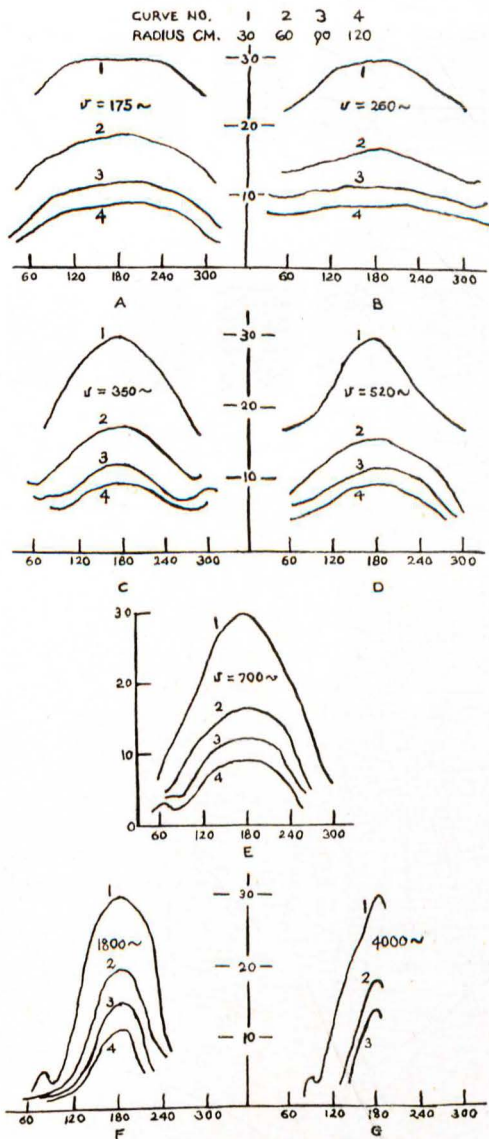
Abb. 21. Richtwirkungsdiagramme des Waldhorns (nach Martin) Fig. 21. Polar diagrams for the French horn (Martin)
