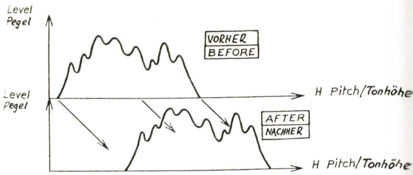
Abb. 9 Fig. 9 Transposition
