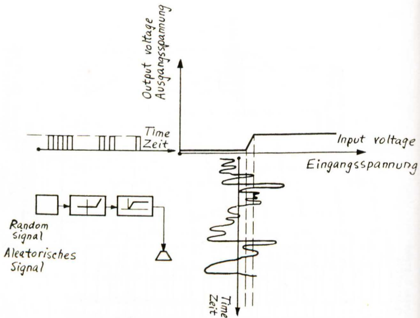
Abb. 6 Der Lieti'sche Amplitudenselektor Fig. 6 Lieti's amplitude selector
