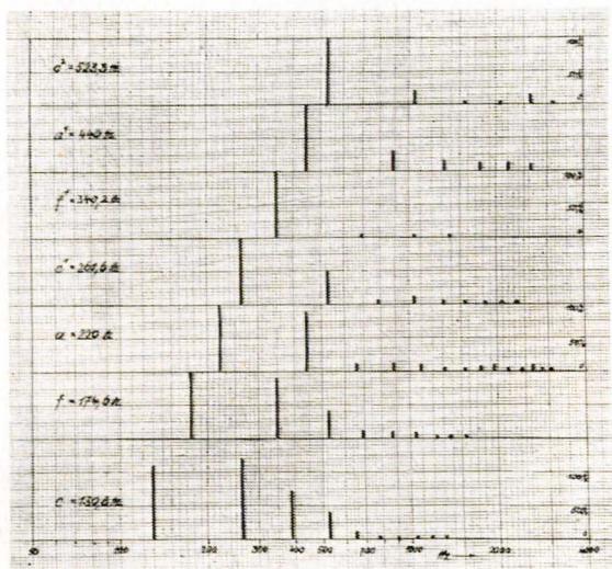
Tafel V Klangspektren Luftschall — gestopft Plate V Sound spectra Airborne sound — stopped
