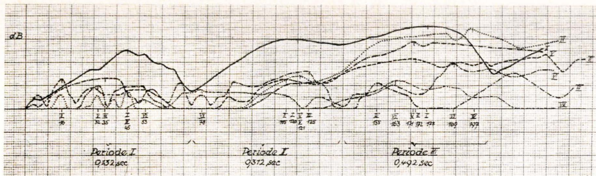
Abb. 16. Einschwingvorgang des B 1 mit Dämpfer (58 Hz). Fig. 16. Attack of muted Bb 1 (58 c/s)
