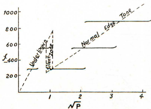
Fig. 1 Schneidentöne in Orgel-Pfeifen
