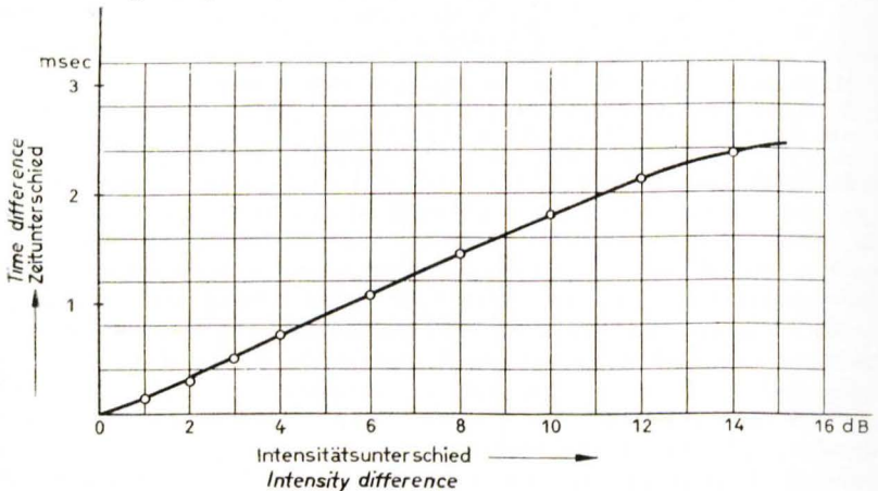
Abb. 1b Zeit-Intensitäts-Äquivalenz an Lautsprechern mit 3,5 m Hörabstand und 3,5 m Basisbreite (bei Sprache, nach Katzfey und Schröder).
