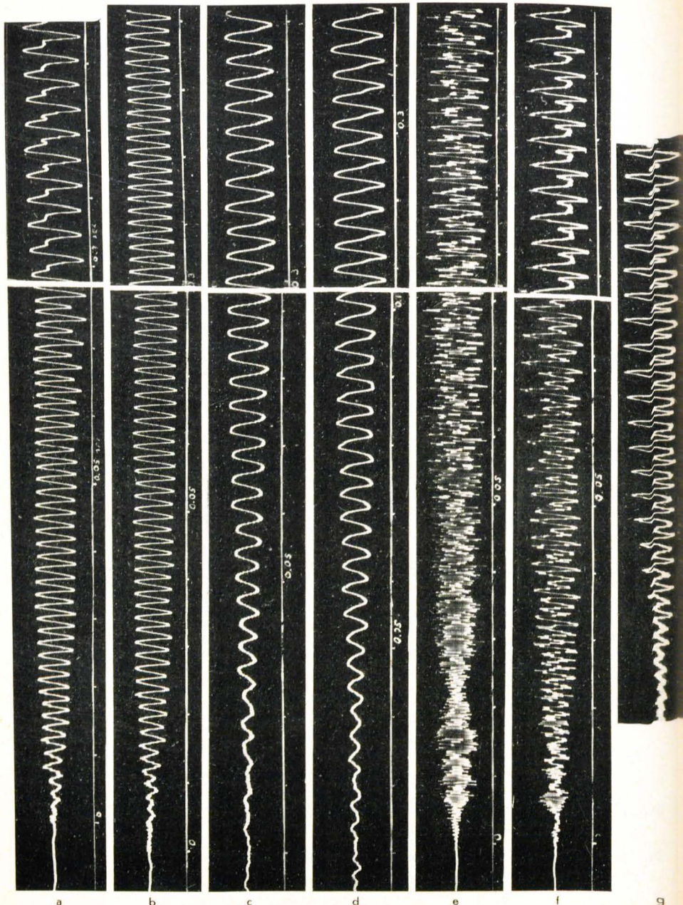
Fig. 3 Die Bildung der Schallwellen in den Orgel-Pfeifen nach Vornahme der verschiedenen Justierungen während des Intonierungs-Vorganges a, b, c, d = Wald-Flöte — e, f, g = Offene Prinzipal-Pfeife.
