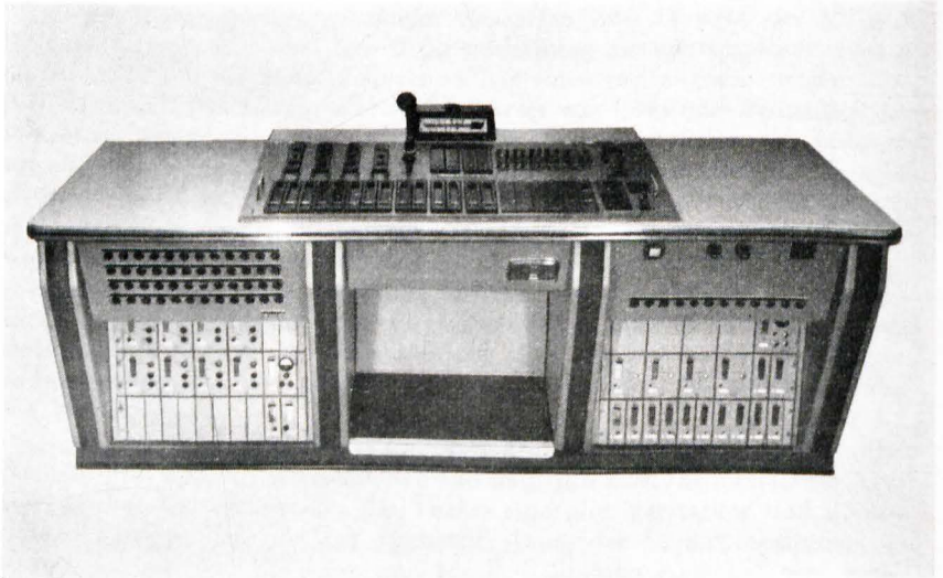
Bild 2 Regietisch für Stereoaufnahmen Fig. 2. Mixer console for stereophonic recording.
