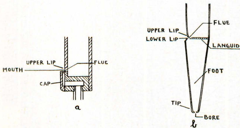
Fig. 2 a. Querschnitt einer hölzernen Orgel-Pfeife der Flöten-Klasse
