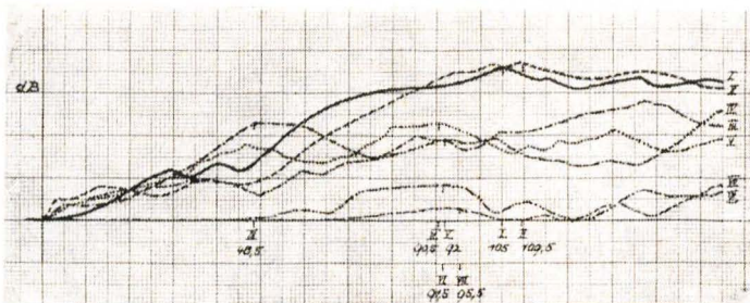
Abb. 14. Einschwingvorgang des offenen B 1 (58 Hz) Fig. 14. Attack transient of open B 1 (58 c/s)
