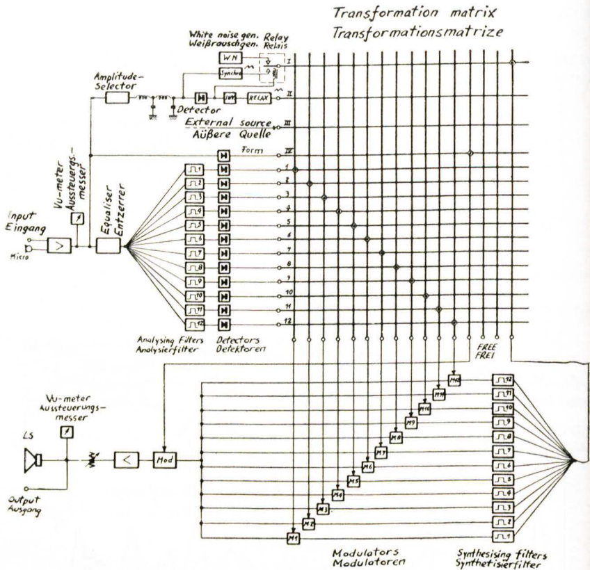
Abb. 10 Fig. 10 Vocoder
