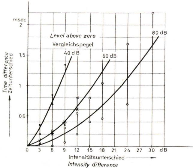
Abb. 1a Äquivalenz von Intensitäts- und Zeitunterschieden direkt am Ohr des Beobachters bei verschiedenen Pegeln. (Nach Deatherage und Hirsch, im Kopfhörer an Tonklicks gemessen).
