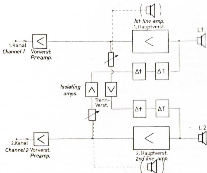
Abb. 3 Schema einer Schaltung zur Steigerung der Raumwirkung bei stereophonischer 2-Kanal-Wiedergabe.
